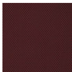
2309 Sagittarius
